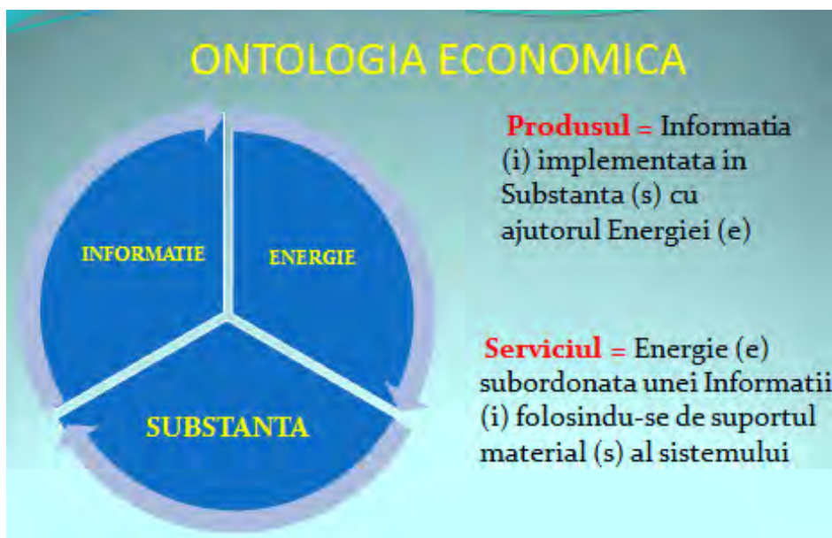
Schema 2. Schema ontologia economică Sursa: Schema elaborată G. Ciobanu și A. Pană în articolul Information and Value in the Scientific Conception of Professor Paul Bran
